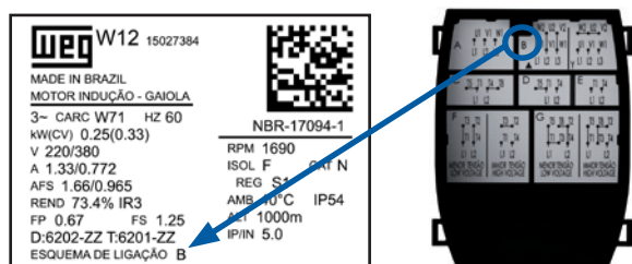
Figura 11 – Esquema da conexão dos cabos de ligação
