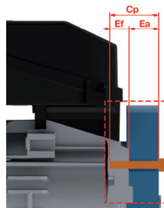
Figura 14 – Comprimento máximo do furo roscado
