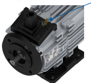
Figura 10 – Terminal de aterramento no hub
