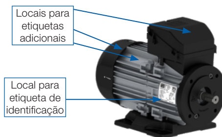
Figura 13 – Localização das etiquetas nos motores W12.
